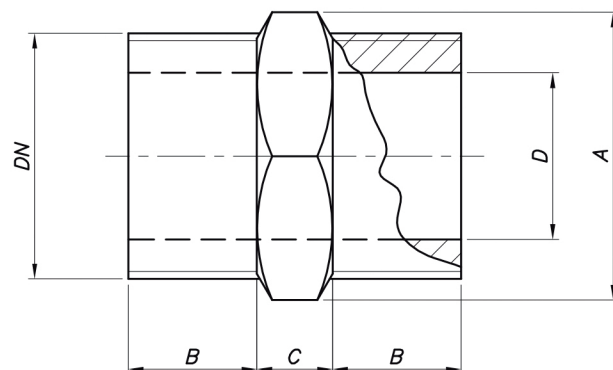
NIPLE SEXTAVADO
