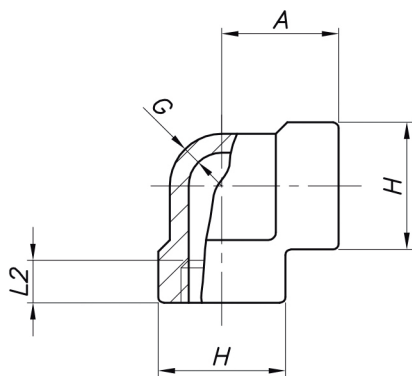
COTOVELO 90°
