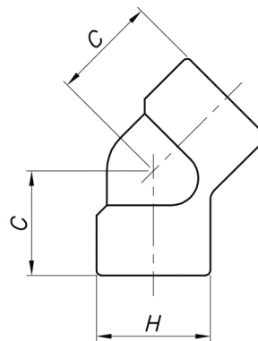
COTOVELO 45°
