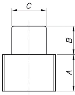
PLUG QUADRADO
