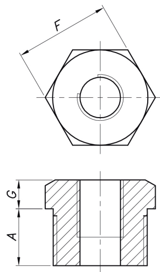
BUCHA SEXTAVADA
